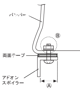
取付状態断面図
