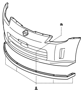
取付参考図
