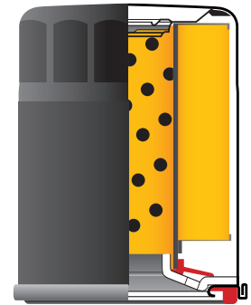
カット図
